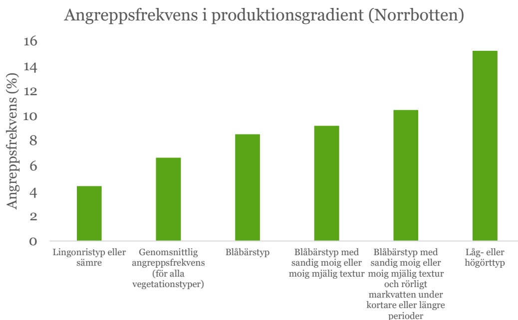
Figur 24. Selektivt konstruerad produktionsgradient och respektive angreppsfrekvenser i Norrbotten. Data är på provyttenivå och avser tallhuvudstammar.
