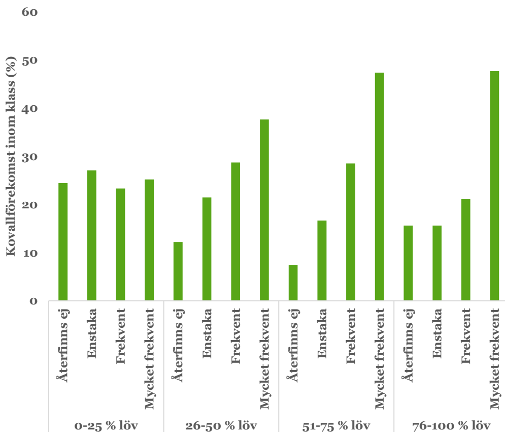
Figur 19. Kovallförekomst i relation till lövandel i Norrbotten, grupperat i klasser om 25 %. Lövandelen är beräknad som summan av bi- och huvudstammar av löv dividerat med summan för alla huvud- och bistammar för alla trädslag. Summan av de individuella kovallförekomsterna inom klass för lövandel är 100 %. Data är beräknat på provytelnivå.
