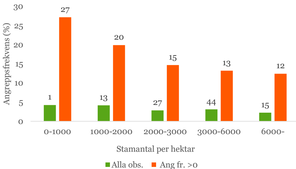
Figur 20. Angreppsfrekvens i relation till stamantal per hektar för alla provytor, samt för de provytor där angreppsfrekvensen var större än noll (Ang. fr. >0). Stamantalet är beräknat som summan av huvud- och bistammar för alla trädslag uppräknat till hektar-nivå. Siffror ovan staplar beskriver andelen observationer inom respektive klass för stamantal. Data är beräknat på provytenivå.
