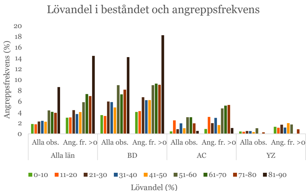
Figur 17. Angreppsfrekvens av törskate i relation till lövandelen i beståndet för hela undersökningen och i länsvis uppdelning (BD = Norrbotten, AC = Västerbotten och YZ är en sammanslagning av Västernorrlands län och Jämtlands län). Data särredovisas för alla bestånd, samt för de bestånd där angreppsfrekvensen var större än noll (Ang. fr. >0). Lövandelen är beräknad som summan av huvud- och bistammar av löv dividerat med summan för alla bi- och huvudstammar för alla trädslag. Data på angreppsfrekvenser avser tallhuvudstammar och är beräknat på beståndsnivå.
