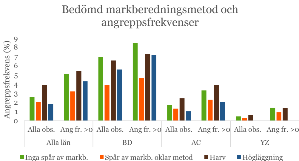
Figur 23. Angreppsfrekvens av törskate i relation till bedömd markberedningsmetod för hela undersökningen och i länsvis uppdelning (BD = Norrbotten, AC = Västerbotten och YZ är sammanslagning av Västernorrlands län och Jämtlands län). Data särredovisas för alla bestånd samt för de bestånd där angreppsfrekvensen var större än noll (Ang. fr. >0). Data avser tallhuvudstammar och är beräknat på beståndsnivå.
